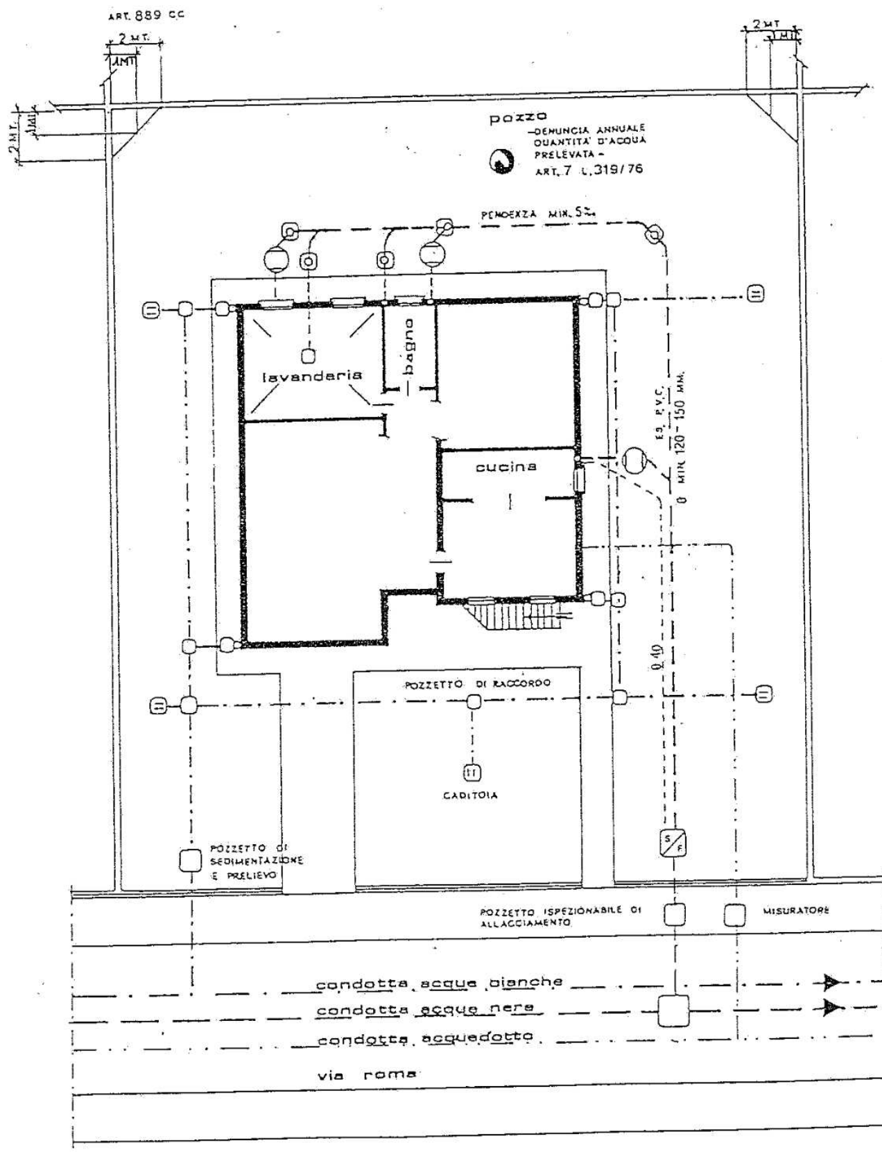
SCHEMA FOGNATURA ACQUE NERE E BIANCHE
